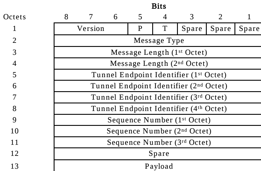
図 3.1-1 GTPv2-C のパケット構成
