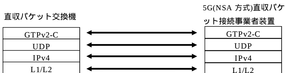
図 1.3-2 直収パケット交換機—5G(NSA 方式)直収パケット接続事業者装置間のプロトコルスタック（GTPv2-C）
