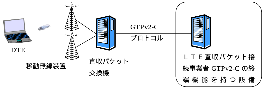
図 1.2-1 システム構成図 (GTPv2-C 接続)
