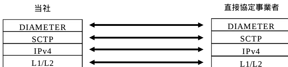
図 1.3-1 プロトコルスタック
