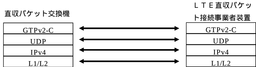
図 1.3-2 直収パケット交換機—LTE 直収パケット接続事業者装置間のプロトコルスタック (GTPv2-C)
