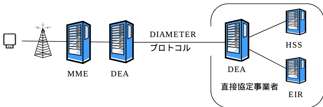
図 1.2-1 システム構成図
