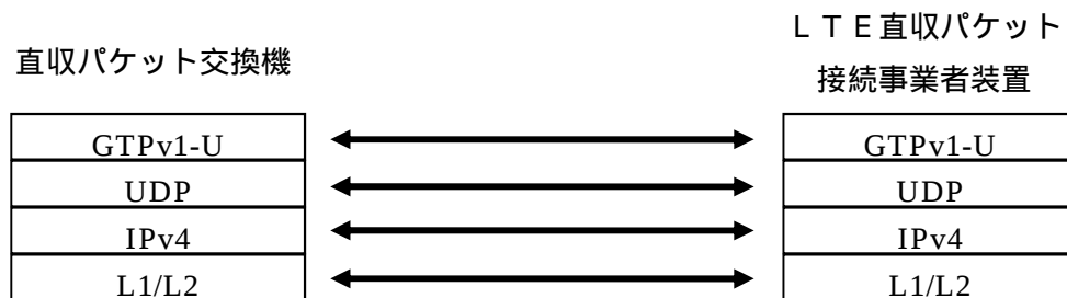
図 4.2-1 直収パケット交換機～LTE直収パケット接続事業者設備間のプロトコルスタック
