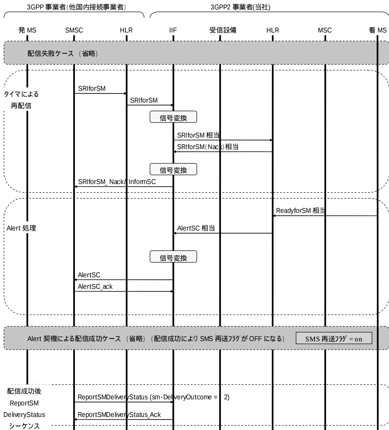
図 2 . 2 - 7 3 G P P ( 他国内接続事業者 ) 3 G P P 2 ( 当社 ) 事業者 ( 基本シーケンス 3 )
