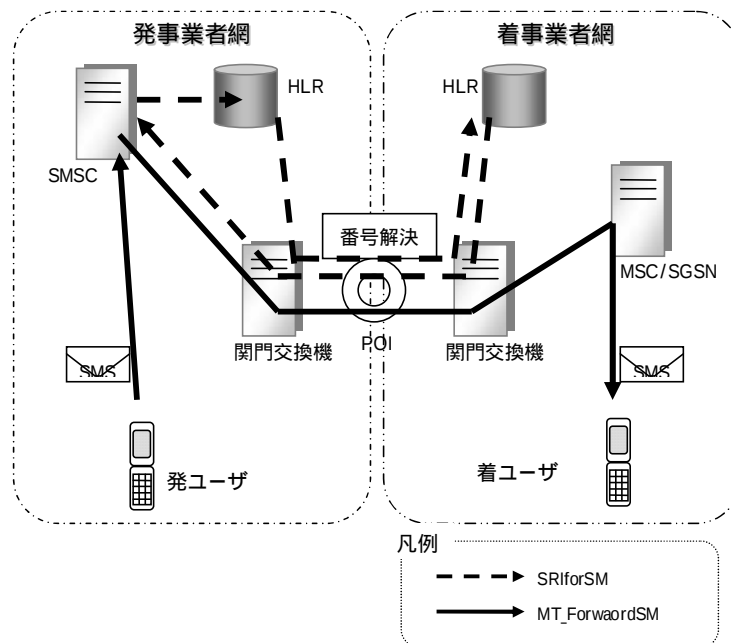
図 2 - 1 国内 S M S 相互接続のイメージ
