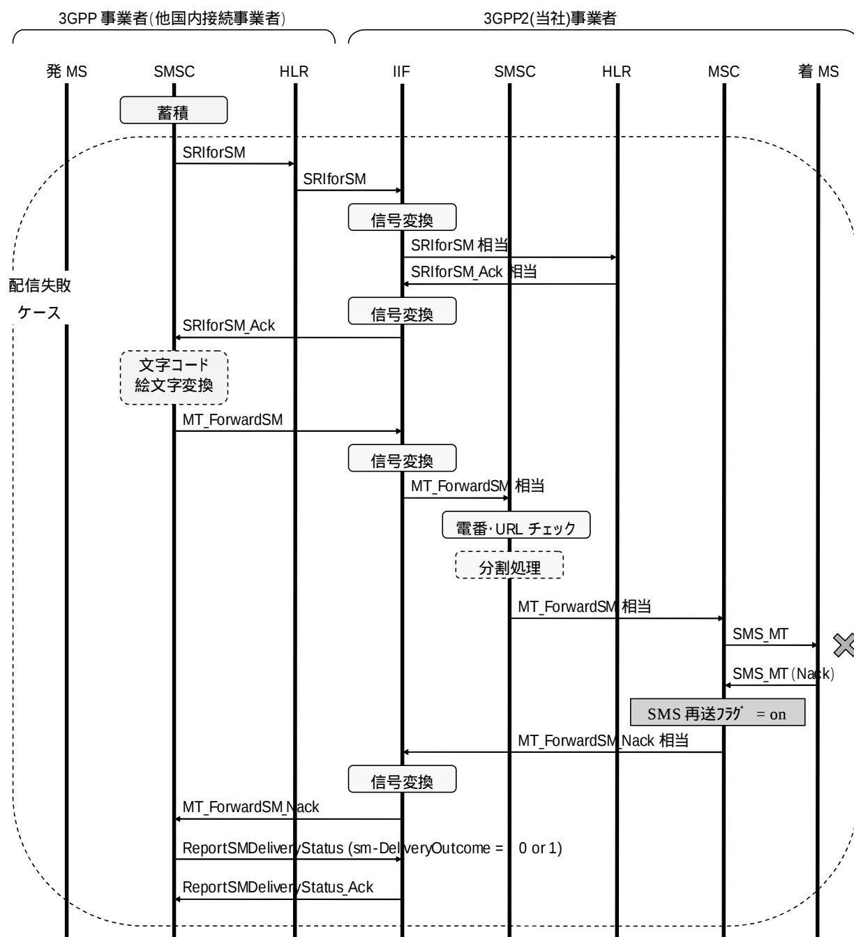
図 2 . 2 - 6 3 G P P ( 他国内接続事業者 ) 3 G P P 2 ( 当社 ) 事業者 ( 基本シーケンス 2 )
