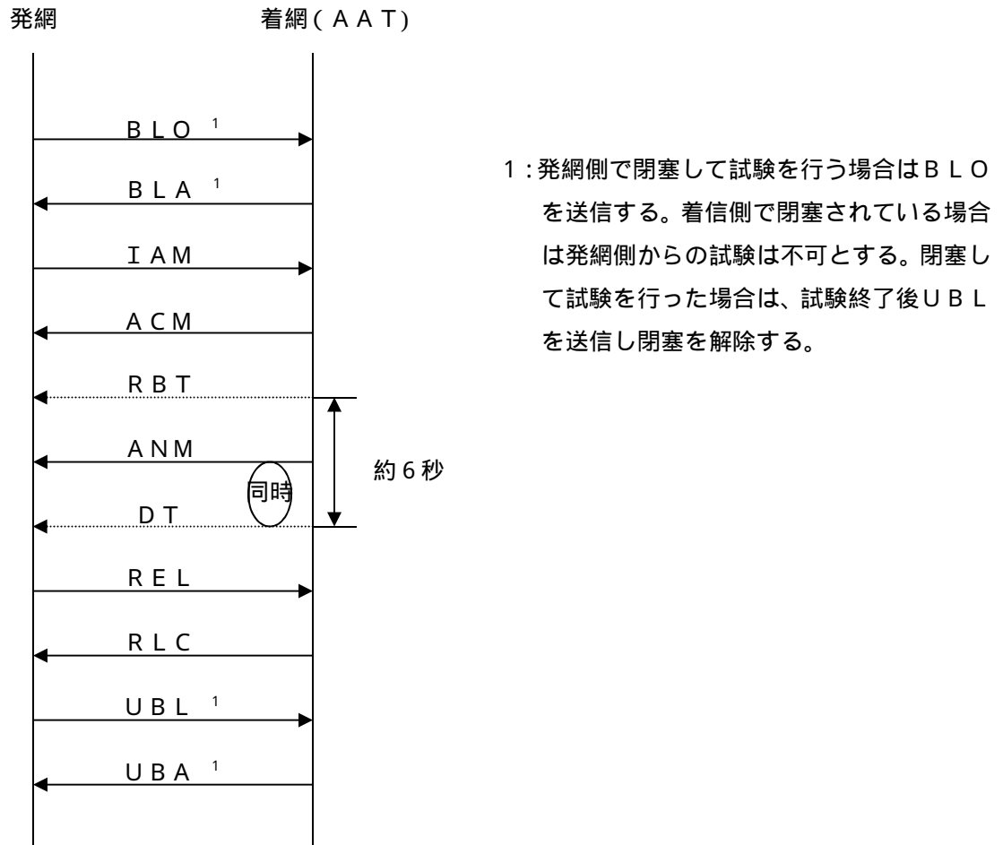
図 5.3-1 課金レート無し，強制切断無し，AAT接続の信号シーケンス
