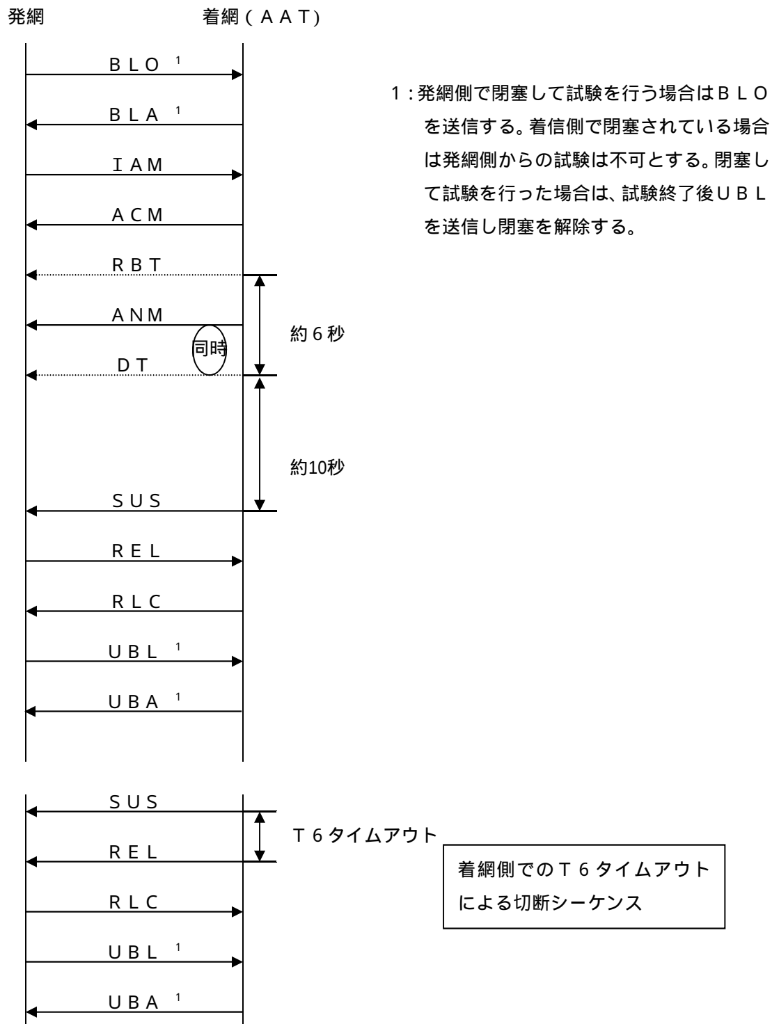
図 5 . 3 - 2 課金レート無し，強制切断有り，AAT接続の信号シーケンス
