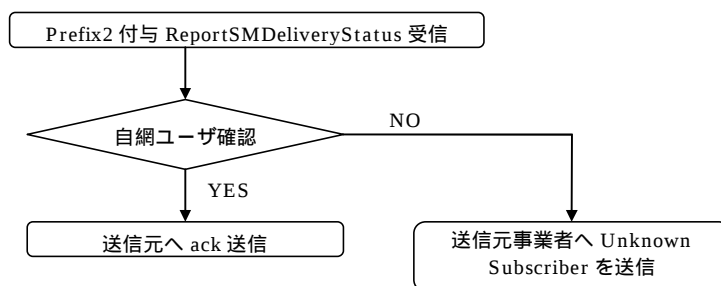
図 2 . 8 - 3 ReportSMDeliveryStatusルーチング判断フロー
