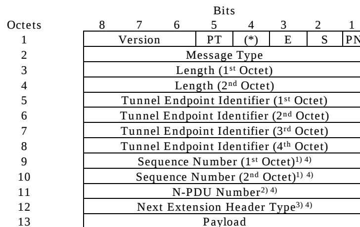
図 6.1-1 GTP-U パケットの構成
