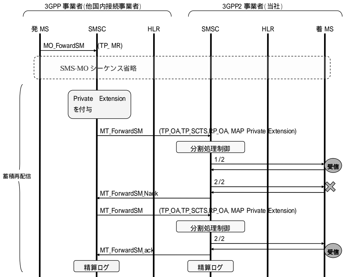
3GPP2 事業者側で 2/2 パート目の配信に失敗し、再配信を行うケース
