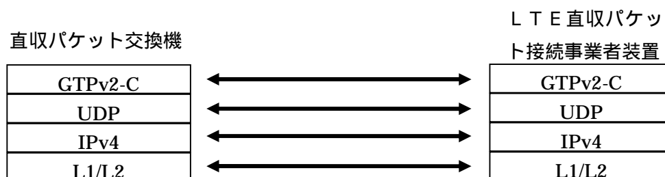
図 1.3-2 直収パケット交換機—LTE 直収パケット接続事業者装置間のプロトコルスタック (GTPv2-C)
