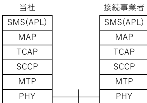
図 2-1 対移動体事業者インタフェース重畳
