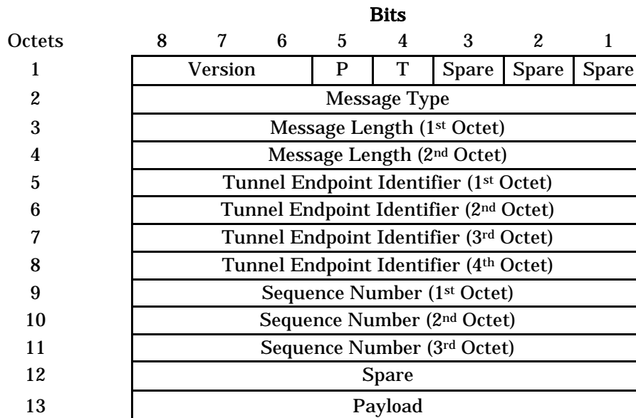
図 3.1-1 GTPv2-C のパケット構成
