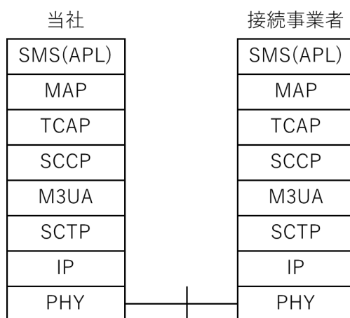
図 2-2 対移動体事業者 (IP) インタフェース重畳
